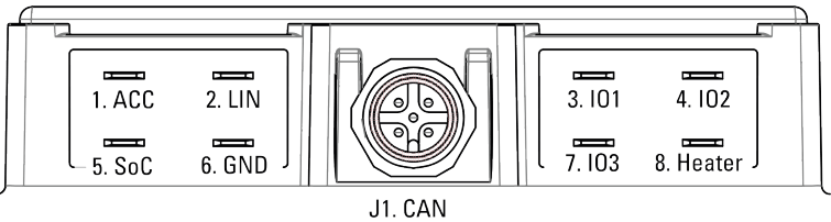
Figure 6. Bornes FASTON. À noter : Les bornes FASTON sont aussi représentées à l'intérieur du couvercle de protection.
